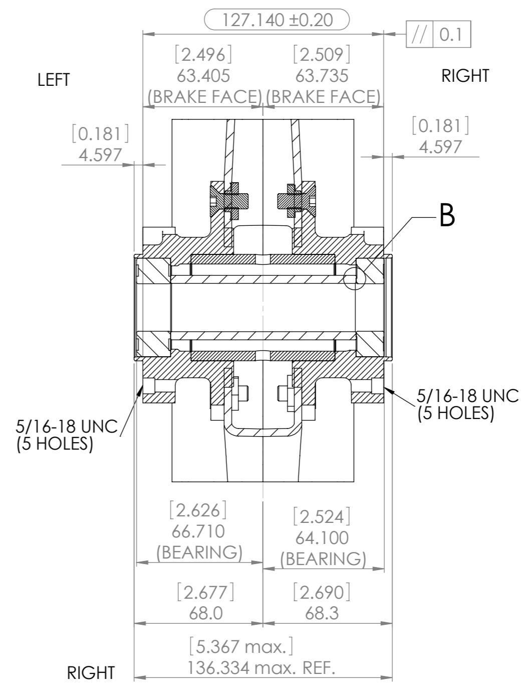
A-A (1 : 2)
