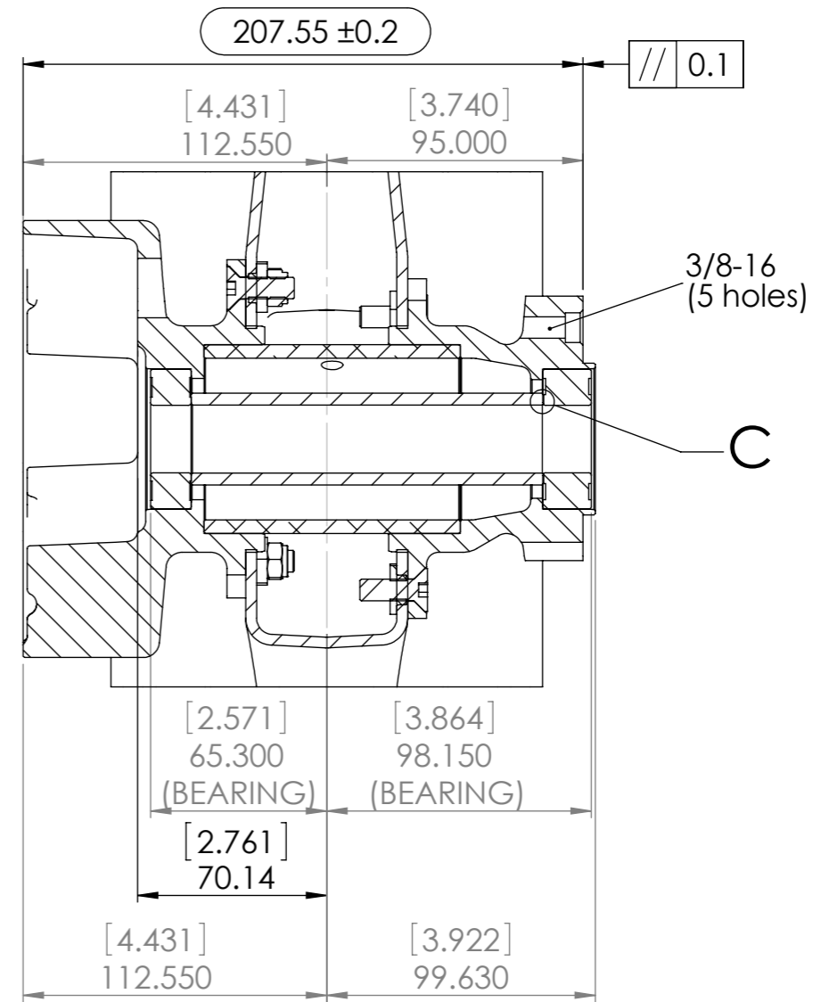
A-A (1 : 2.5)
