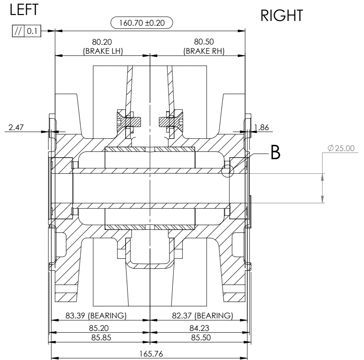
A-A (1 : 2)
