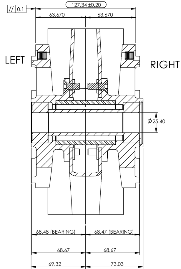
A-A (1 : 2)
